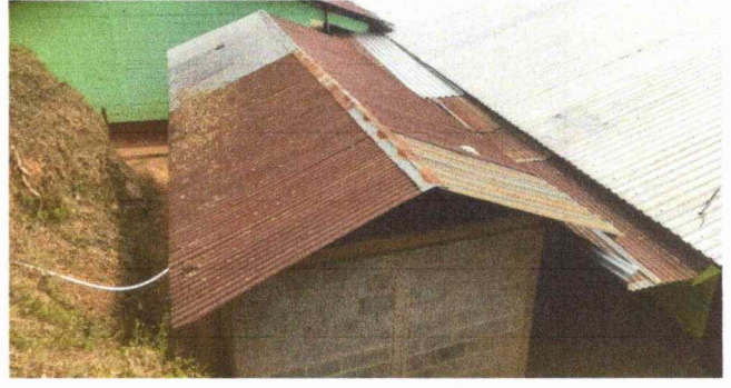
Foto 4: Vista de la cubierta de la cocina a sustituir junto con la estructura.
